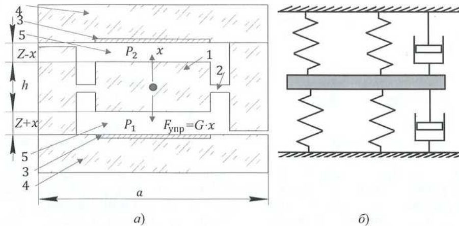
Рисунок 1 – Устройство для осуществления нового способа измерения абсолютного давления газа: а – поперечный разрез, где, проводящая подвижная пластина-осциллятор - 1, упругие подвесы пластины-осциллятора с коэффициентом упругости равным G_m . - 2, электроды - 3, пластины из диэлектрического материала - 4, измерительные газовые зазоры - 5; б - эквивалентная схема «пружинного» маятника
