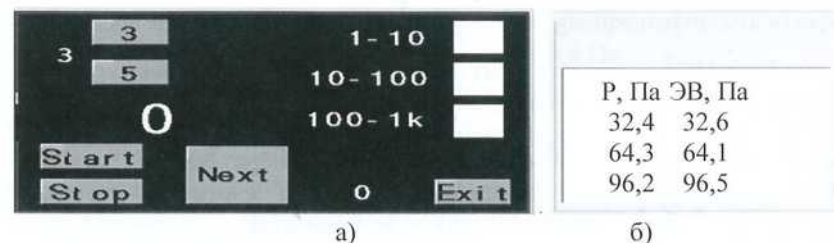
Рисунок 4 – Окна управления: а – процессом автоматической калибровки; б – протоколирования результатов измерений
